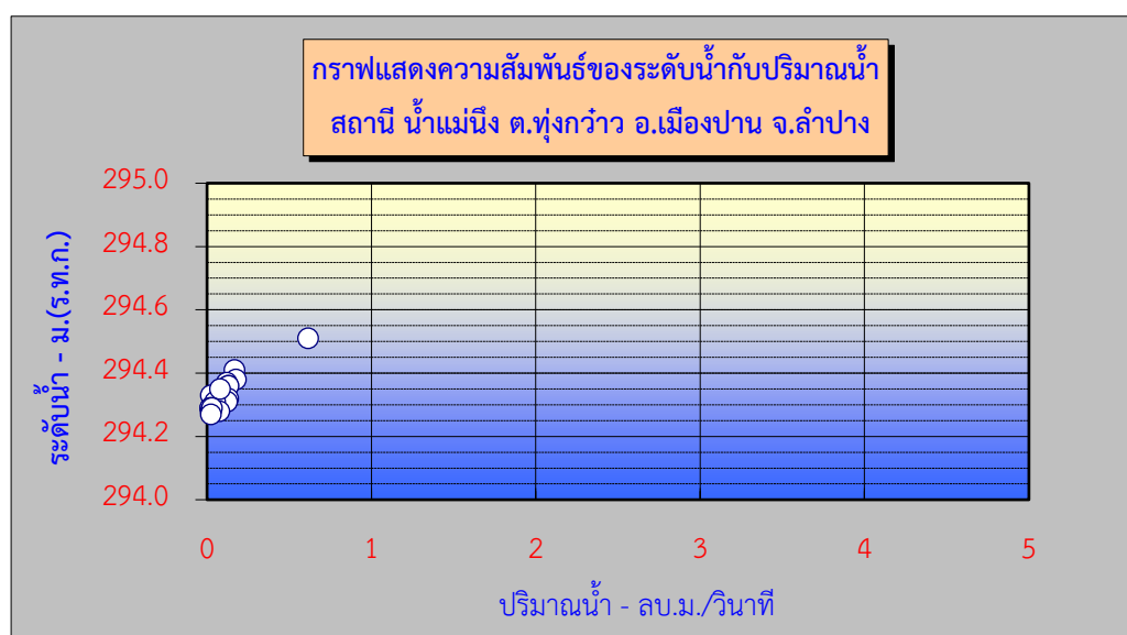
รูปที่ 13 กราฟแสดงความสัมพันธ์ของระดับน้ำกับปริมาณน้ำสถานี ห้วยแม่เนื่อง บ้านป่าเวียง อ.เมืองปาน จ.ลำปาง
